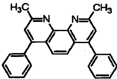
Vasocuproin:
